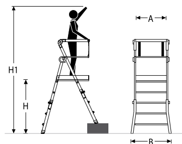
Podwyższona krawędź zabezpieczająca przed upadkiem towarów. Raised edge to prevent materials from falling.
